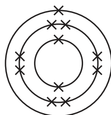
sodium atom
