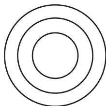
sodium ion
